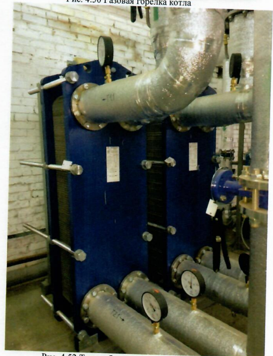
Рис. 4.52 Теплообменное оборудование
