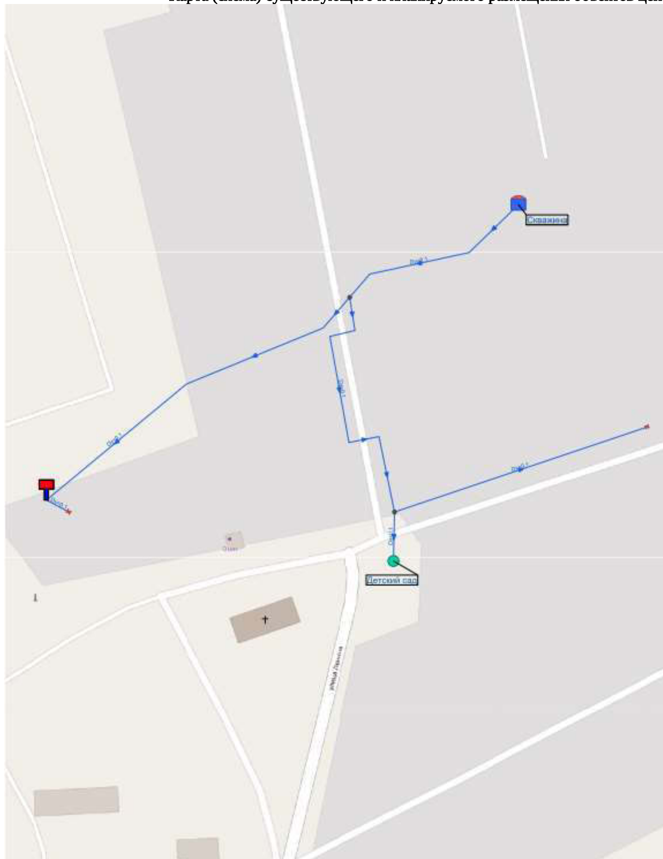
Карта (схема) существующего и планируемого размещения объектов централизованных систем горячего водоснабжения, холодного водоснабжения деревни Ключи
