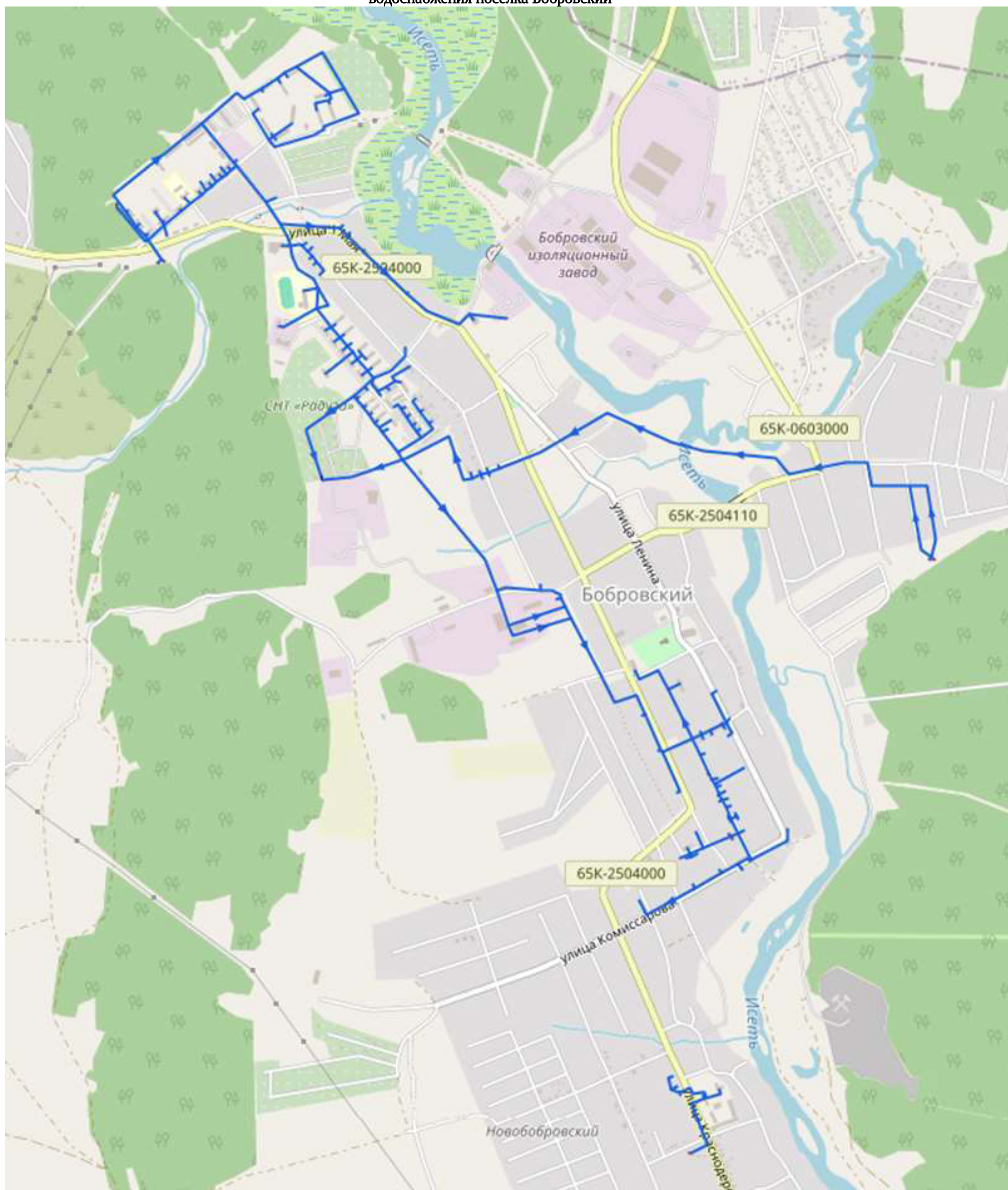
Карта (схема) существующего и планируемого размещения объектов централизованных систем горячего водоснабжения, холодного водоснабжения поселка Бобровский
