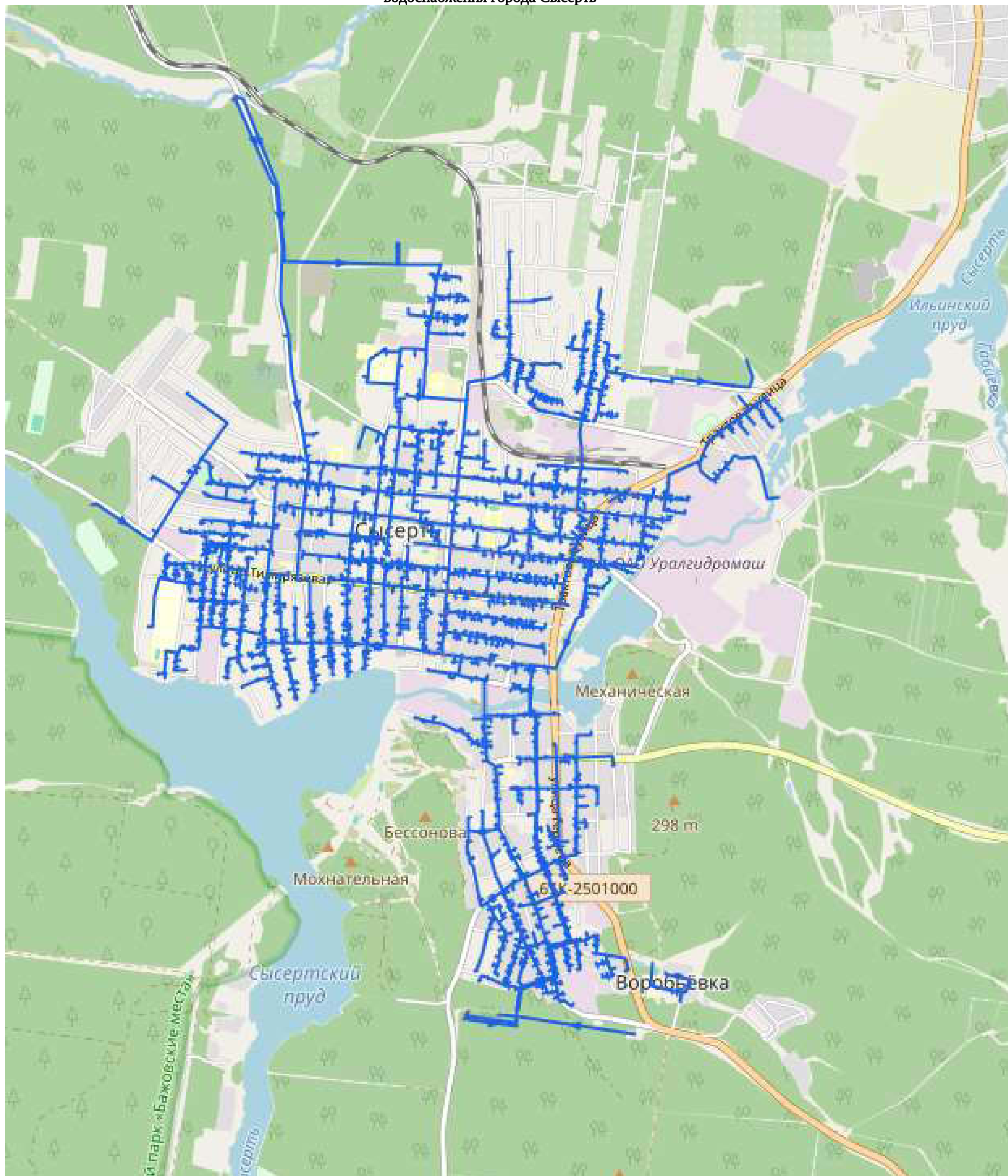
Карта (схема) существующего и планируемого размещения объектов централизованных систем горячего водоснабжения, холодного водоснабжения города Сысерть
