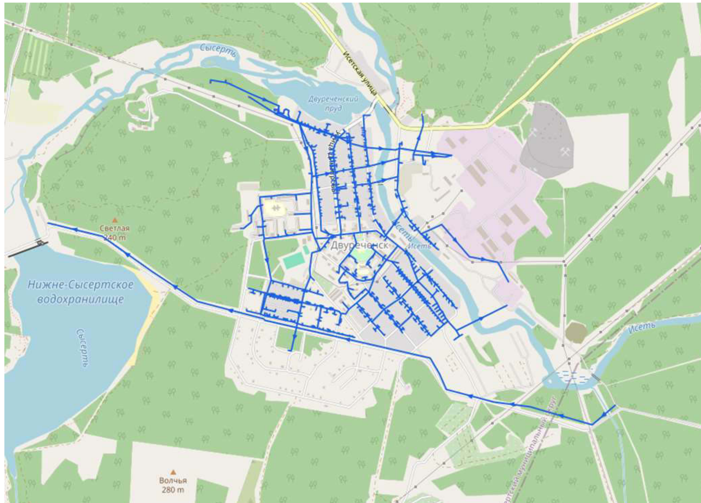
Карта (схема) существующего и планируемого размещения объектов централизованных систем горячего водоснабжения, холодного водоснабжения поселка Двуреченск
