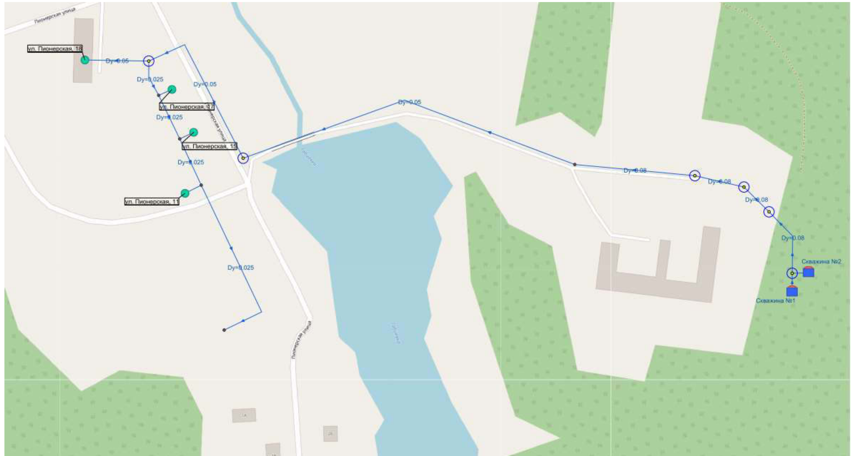
Карта (схема) существующего и планируемого размещения объектов централизованных систем горячего водоснабжения, холодного водоснабжения поселка Школьный
