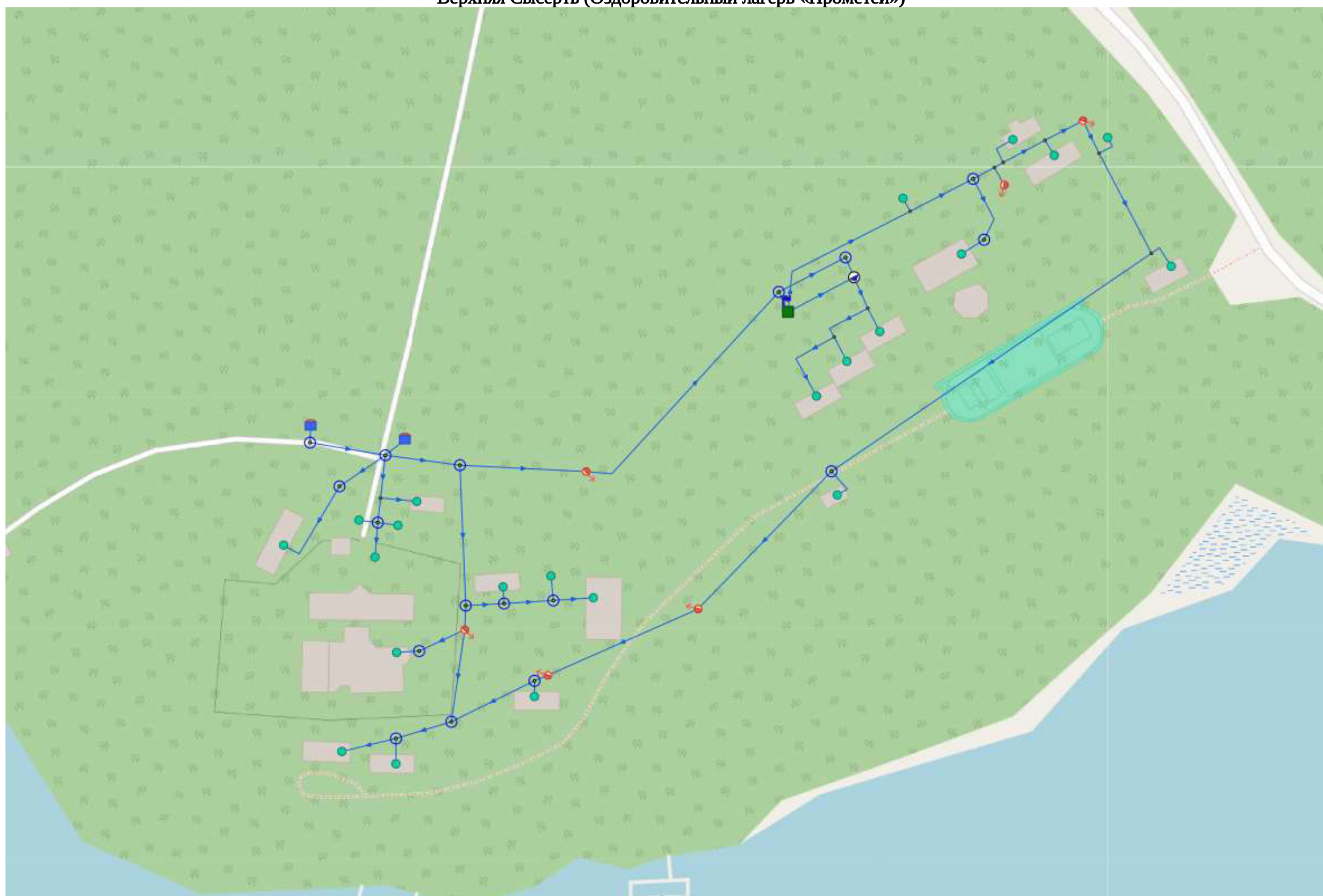
Карта (схема) существующего и планируемого размещения объектов централизованных систем горячего водоснабжения, холодного водоснабжения Верхняя Сысерть (Оздоровительный лагерь «Прометей»)
