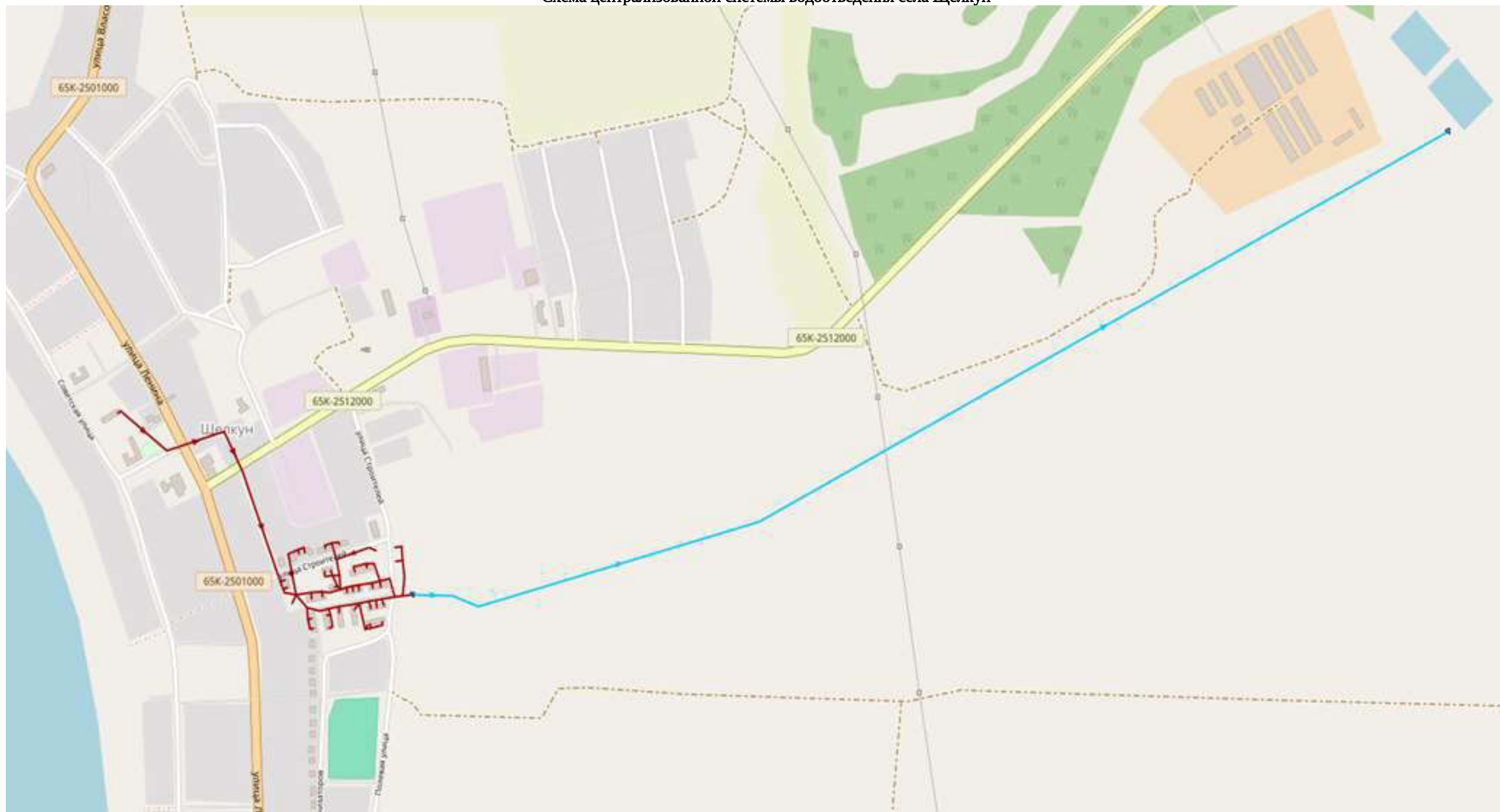
Схема централизованной системы водоотведения села Щелкун
