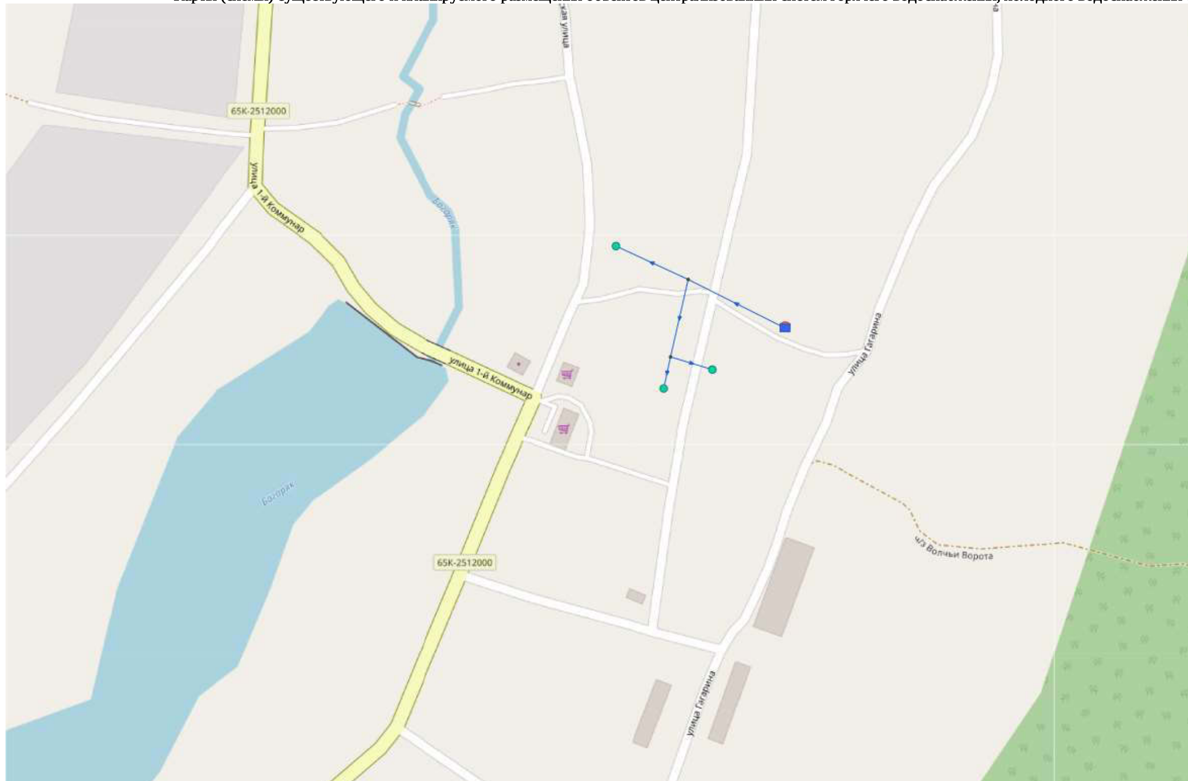
Карты (схемы) существующего и планируемого размещения объектов централизованных систем горячего водоснабжения, холодного водоснабжения села Авериное
