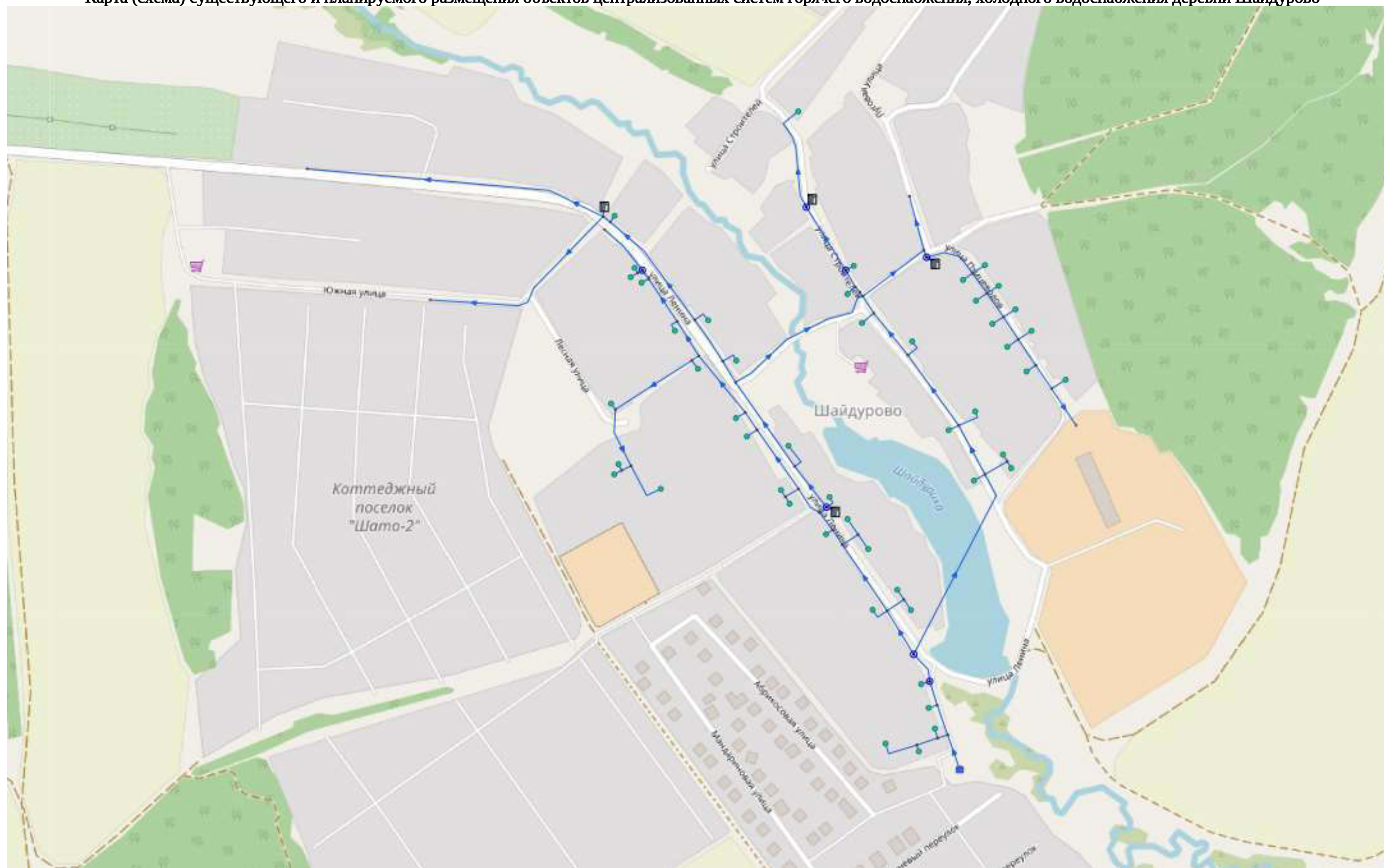
Карта (схема) существующего и планируемого размещения объектов централизованных систем горячего водоснабжения, холодного водоснабжения деревни Шайдурово
