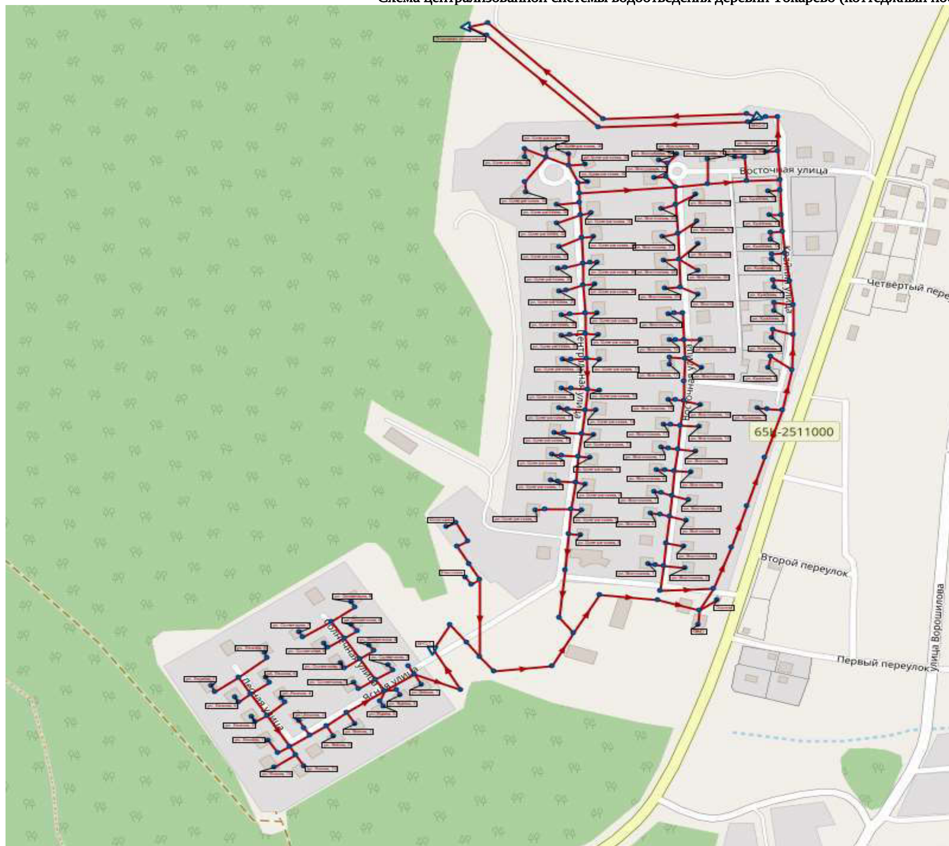
Схема централизованной системы водоотведения деревни Токарево (коттеджный поселок «Газовик»)
