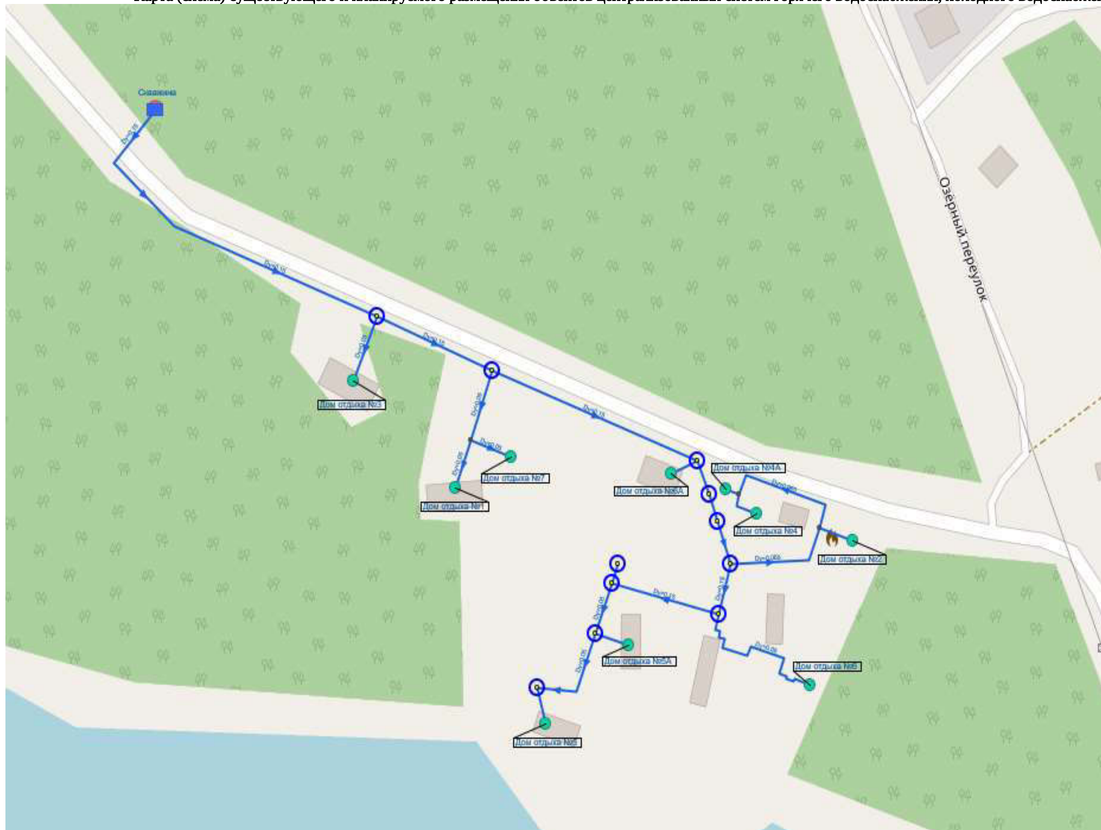
Карта (схема) существующего и планируемого размещения объектов централизованных систем горячего водоснабжения, холодного водоснабжения поселка Верхняя Сысерть
