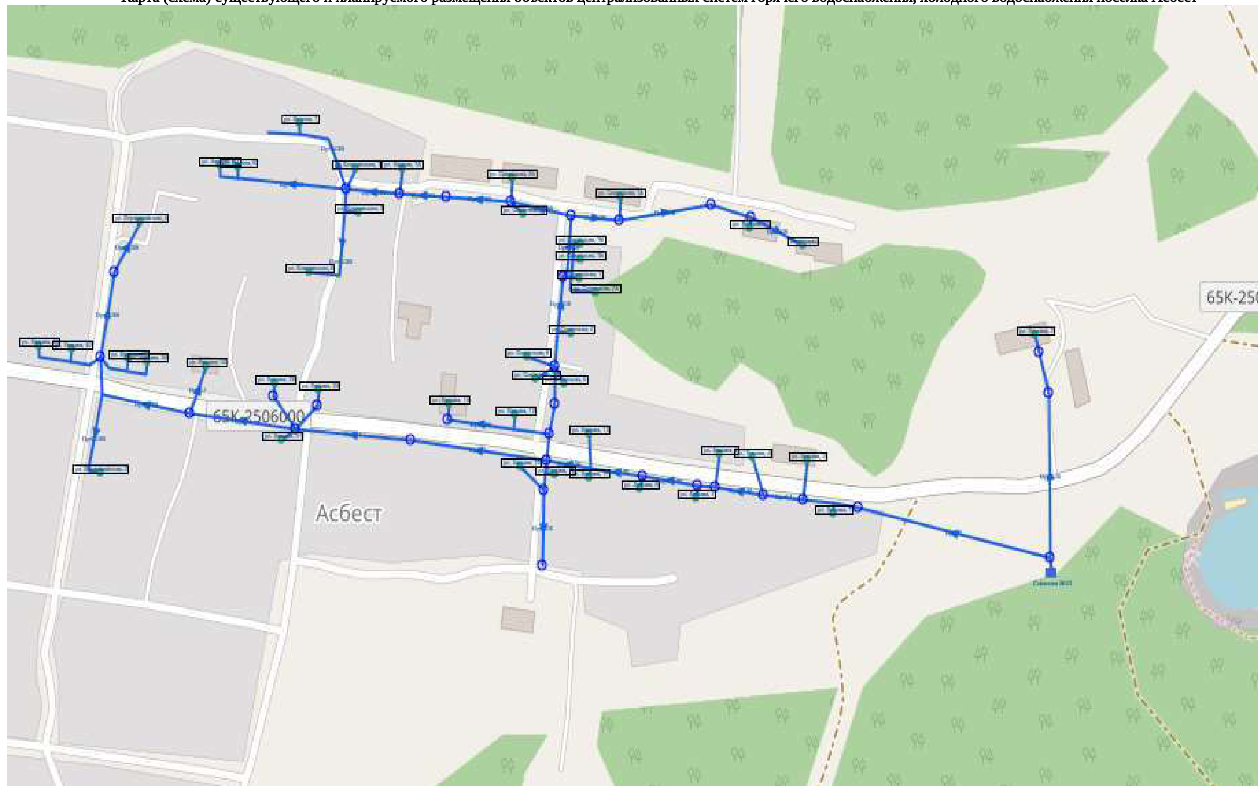
Карта (схема) существующего и планируемого размещения объектов централизованных систем горячего водоснабжения, холодного водоснабжения поселка Асбест
