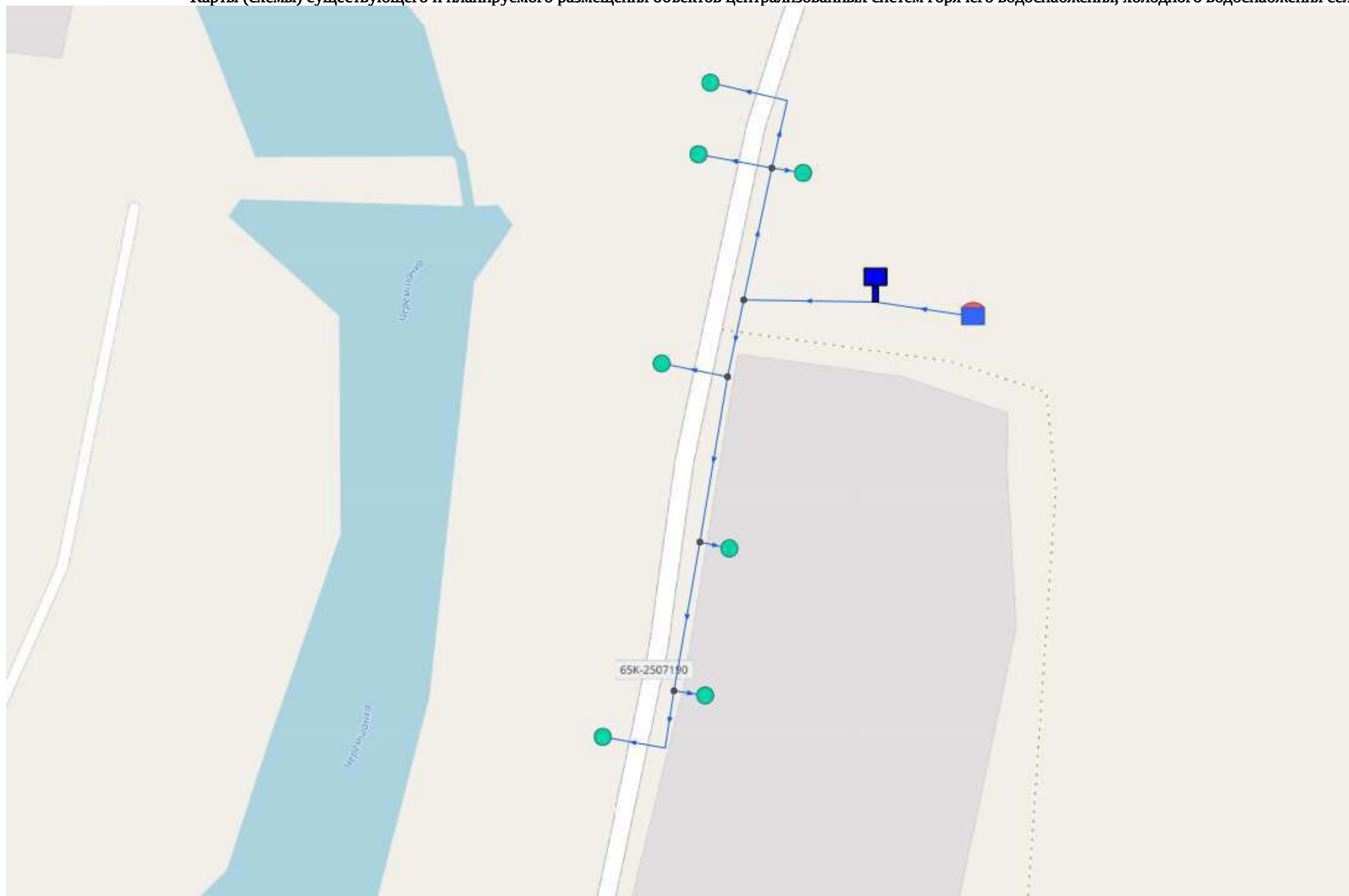
Карты (схемы) существующего и планируемого размещения объектов централизованных систем горячего водоснабжения, холодного водоснабжения села Абрамово
