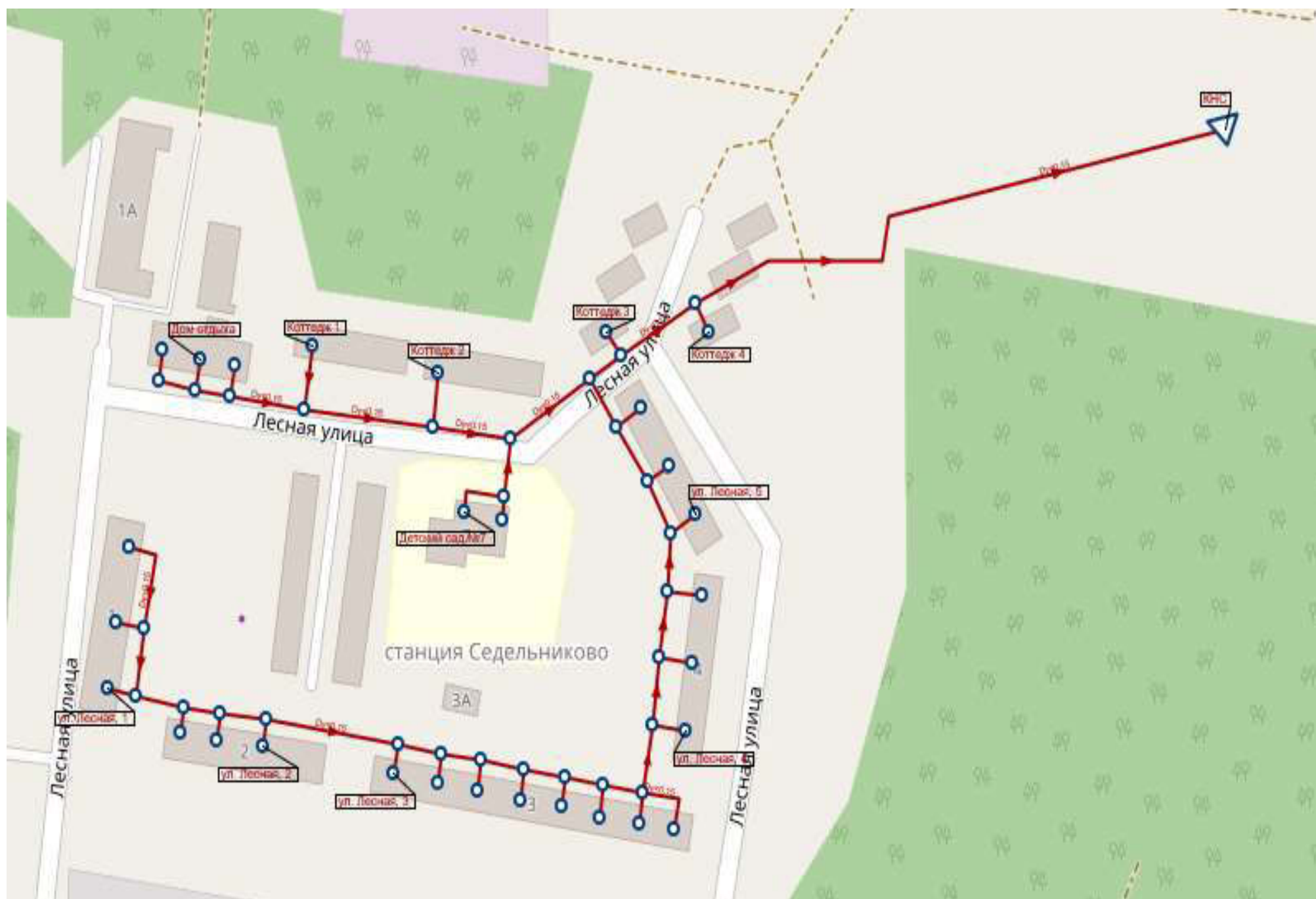
Схема централизованной системы водоотведения улицы Лесная деревни Большое Седельниково
